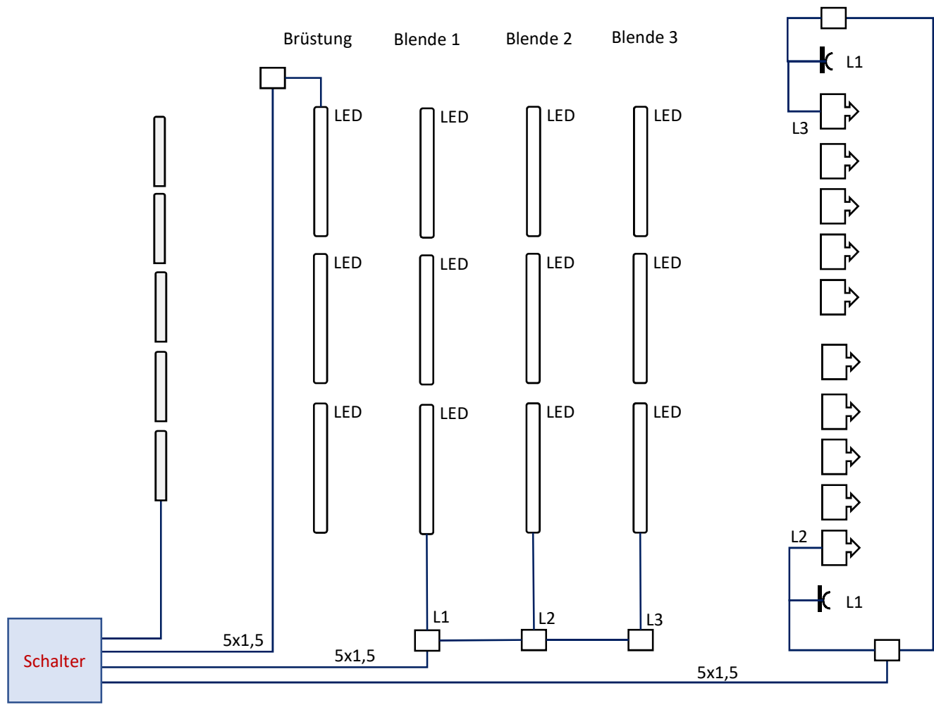
SSV Hilfsbach – Standbeleuchtung 25m © 2018 ITBS
